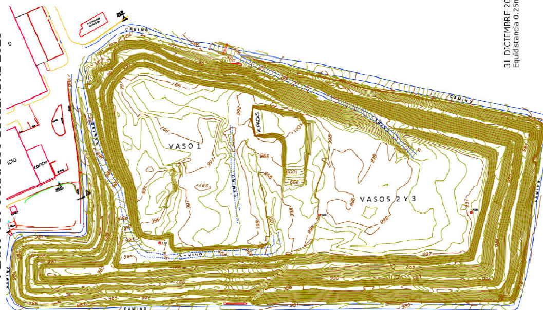
PLANO TOPOGRÁFICO DICIEMBRE 2023
